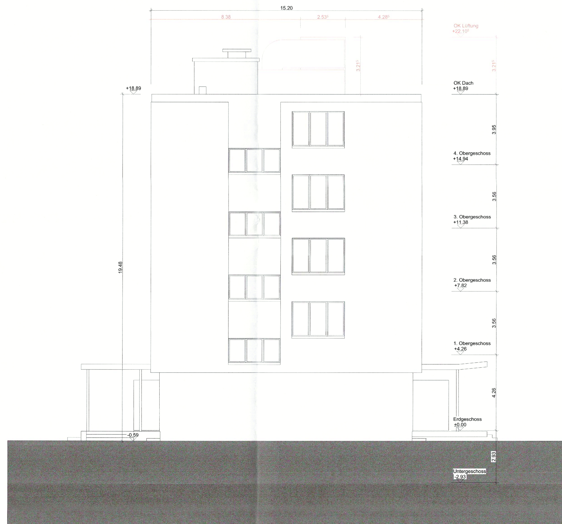
Fassade Ost
