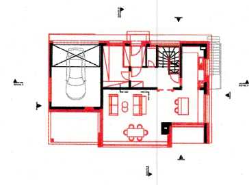
Referenz Grundriss EG
