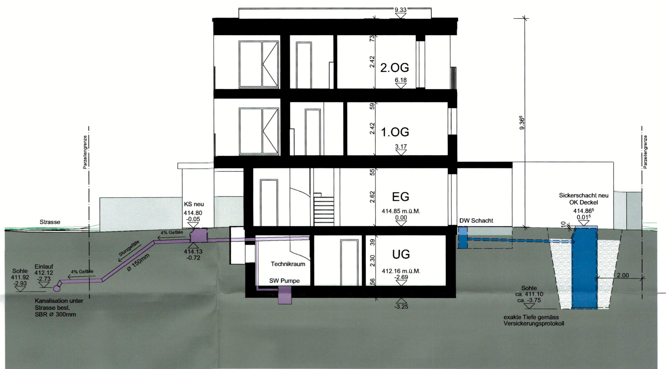
QS/02 Schnitt mit Werkleitungen 1:100
