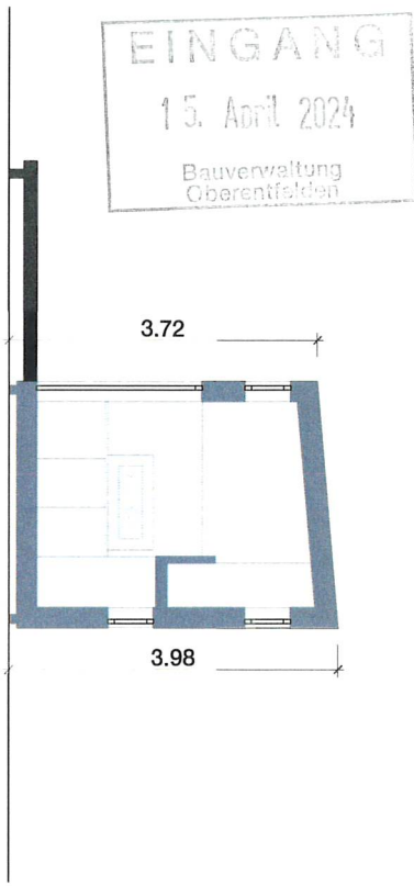
Grundriss Obergeschoss, 1:100
