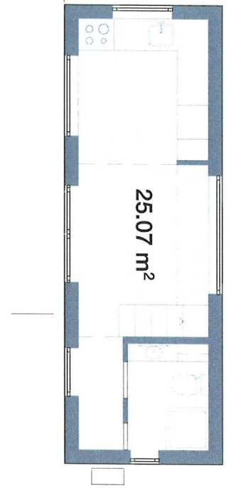
Grundriss Erdgeschoss, 1:100
