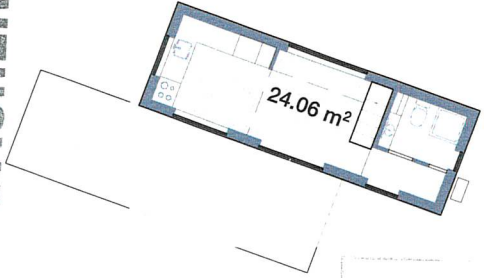
Grundriss Erdgeschoss, 1:200
